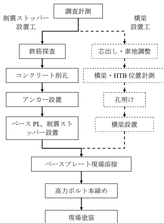
図-10.1 制震ストッパーの施工フロー
