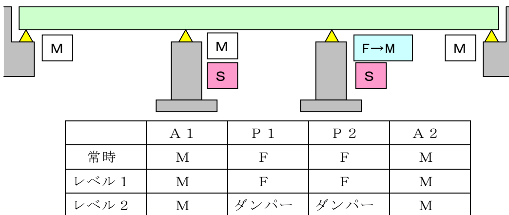
図解-11.6 多点固定構造 2
