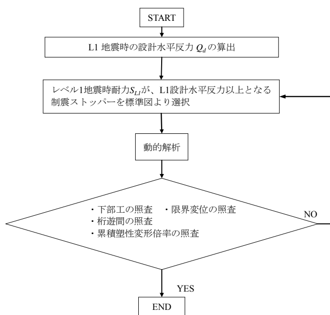
図-7.1 制震ストッパーの設計フロー
