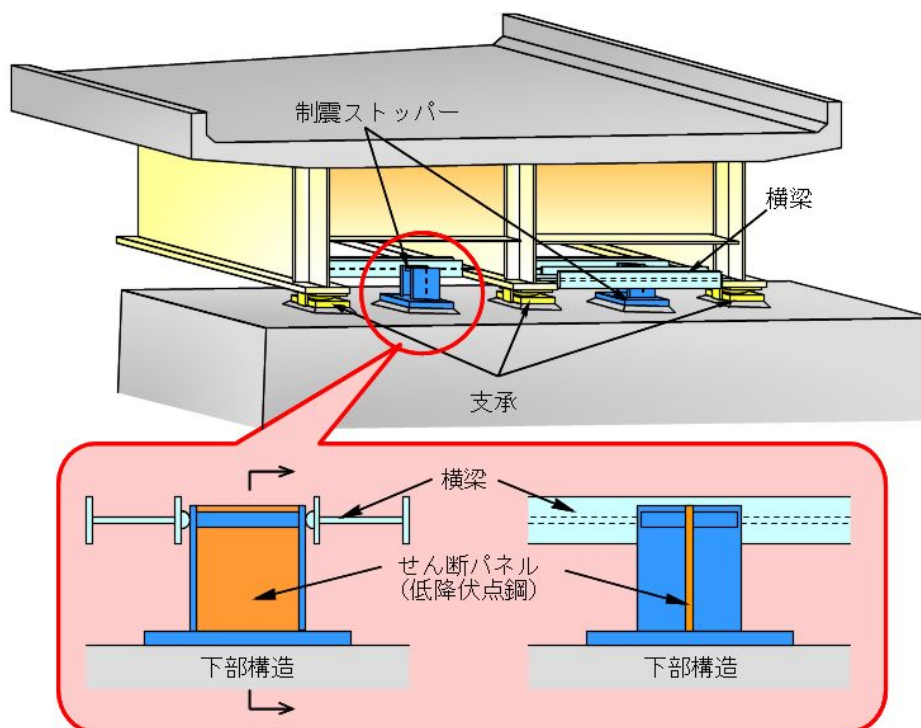
図解-2.1 制震ストッパーの設置イメージ
