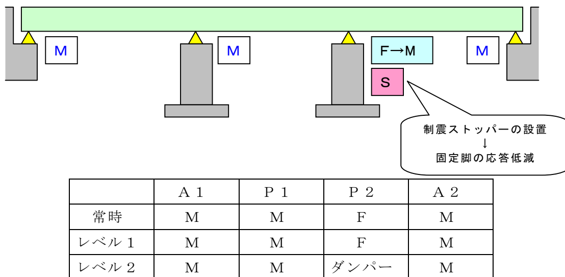
図.解-11.3 橋脚設置例
