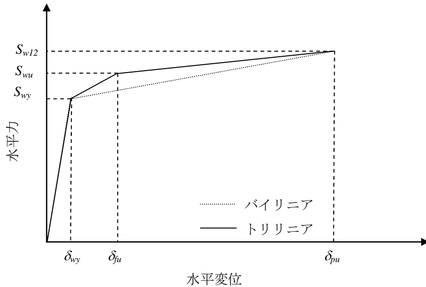
図解-8.1 制震ストッパーの設計曲線
