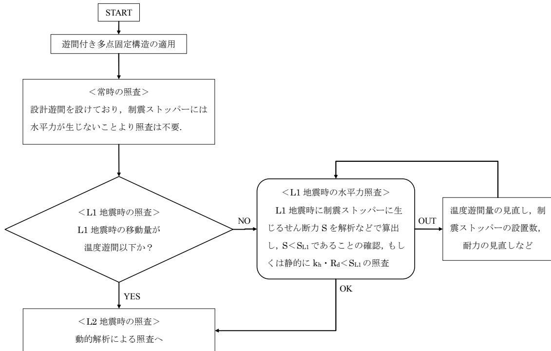
図解-11.10 遊間付き多点固定構造の照査フロー
