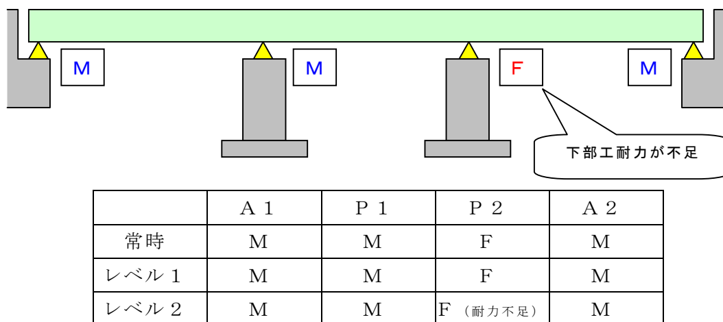
図.解-11.1 既設橋の支承条件
