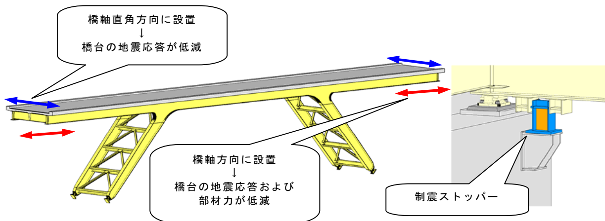
図解-11.12 πラーメン橋への適用例
