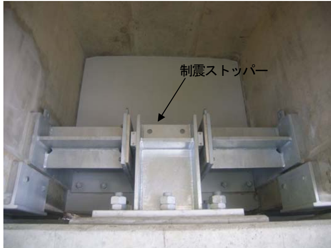
写真-4 PC橋の橋軸直角方向に設置
