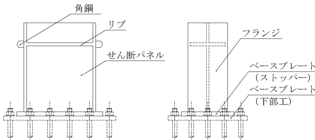
図-3.1 制震ストッパーの構造
