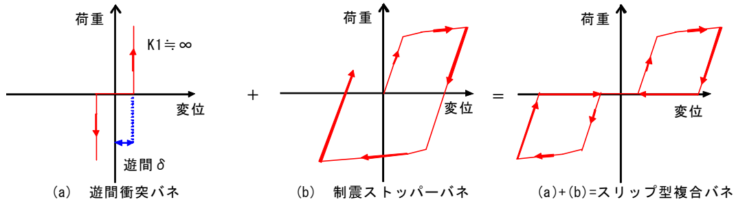
図解-11.9 遊間を考慮した制震ストッパーのモデル化
