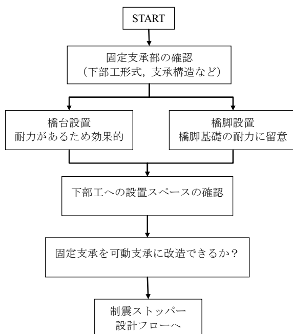
図解-7.1 制震ストッパーの設置フロー
