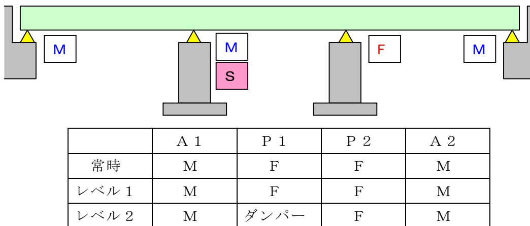
図解-11.5 多点固定構造 1
